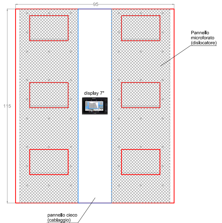
PARTICOLARE ANTA VENTILATORI
